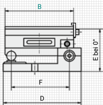
С электропостоянными плитами (EP), P = 4 мм
